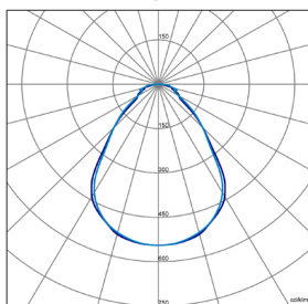
LPRISMA-M/E-IP54-55W
