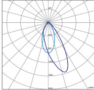
RTK/ASYM (D)-1500-115W
