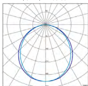
P/OPAL/L-IP65-55W
